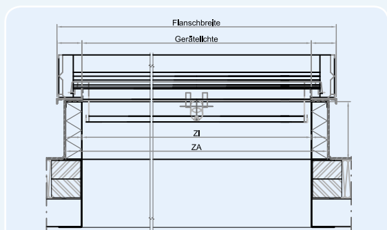
Querschnitt (Sockelmontage mit LB)
