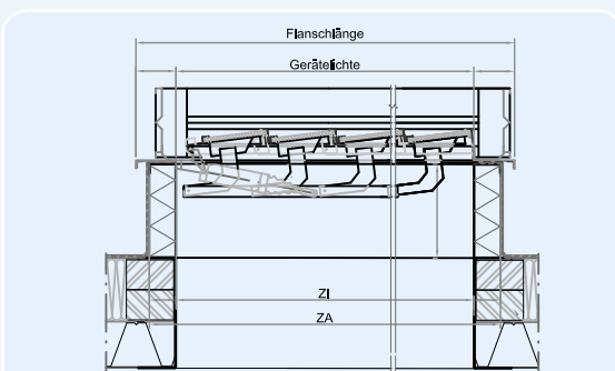
Längsschnitt (Sockelmontage mit LB)
